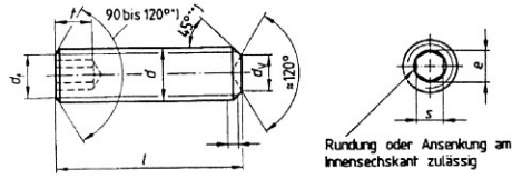
916 - MIT RINGSCHNEIDE
