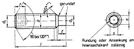
915 - MIT ZAPFEN
