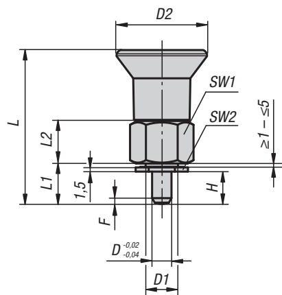
Provedení A bez aretační drážky
