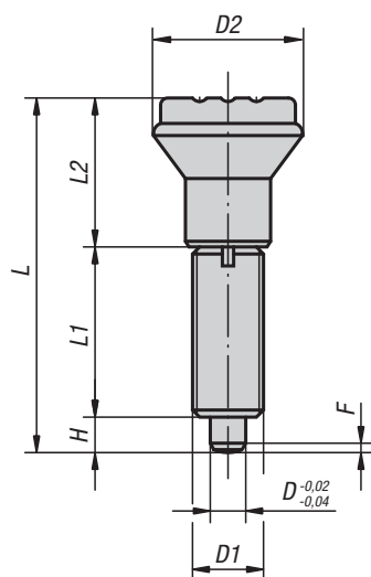
Provedení G bez protimatici
