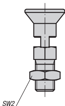
Provedení D s aretační drážkou, s protimaticí
