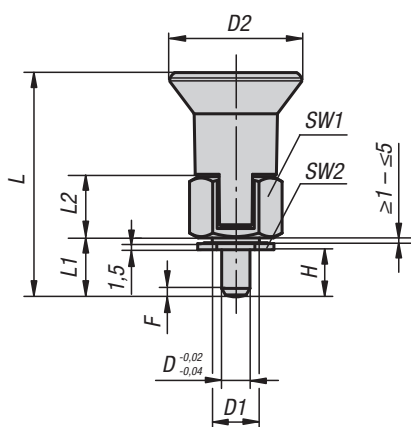
Provedení C s aretační drážkou
