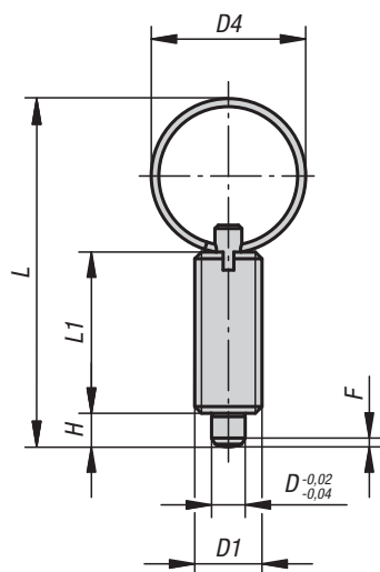
Provedení T bez protimaticí
