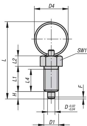
Provedení R bez protimatice
