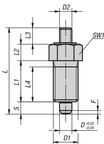
Provedení E se závitovým kolíkem bez protimatice
