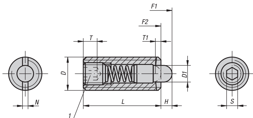
Opěrka zobrazená v celkovém řezu
